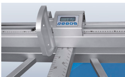
Métrieologie magnétique comme solution personnalisée dans une scie circulaire à format
