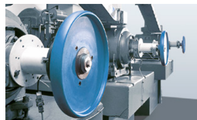
Mesure de vitesse de rotation dans les applications très exigeantes quant aux chocs et aux vibrations
