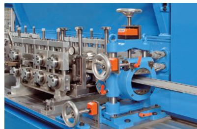
Réglage précis d'une machine à travailler la tôle
